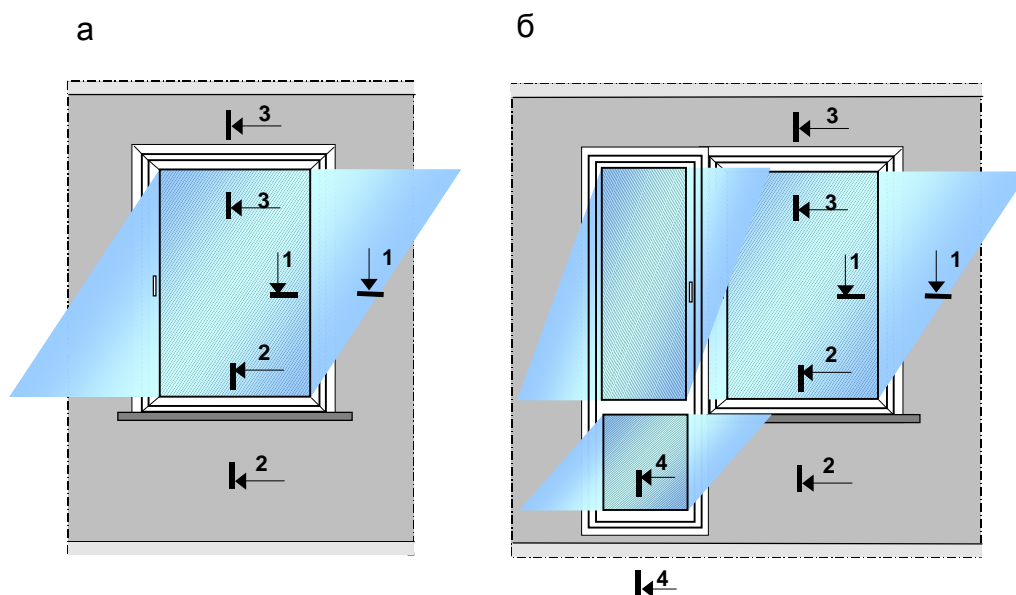
Рисунок Г.1– Схема расположения сечений для проверки температурного режима узлов примыканий оконных блоков к наружным стенам: а – оконного блока; б – балконной двери
