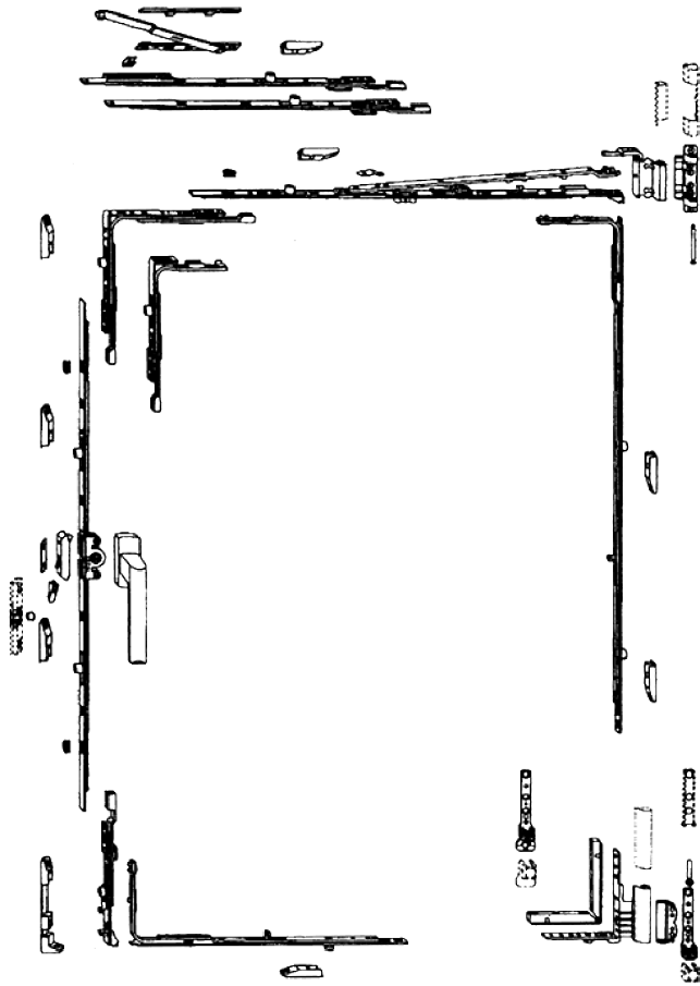
Рисунок Б.3 Устройство поворотно-откидное
