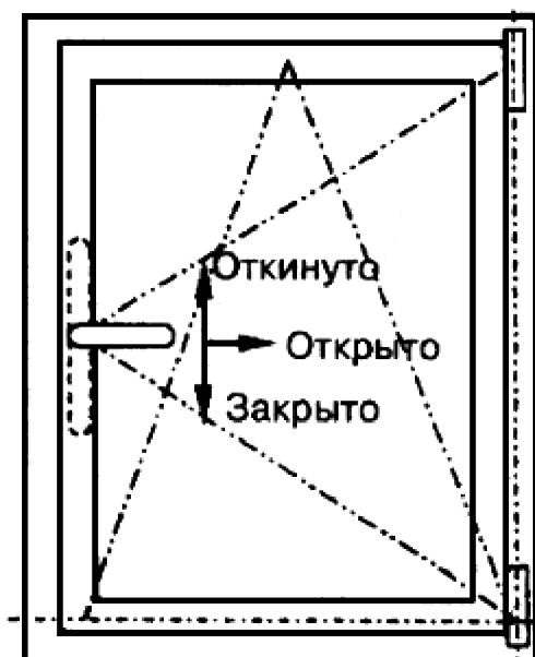
Рисунок А.3 Устройство поворотно-откидное
