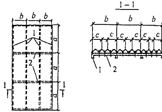
1 - продольные ребра; 2 - поперечные ребра
