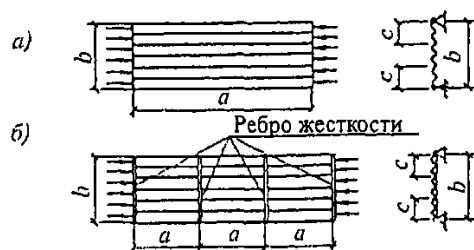
а - без поперечных ребер жесткости; б - с поперечными ребрами жесткости
