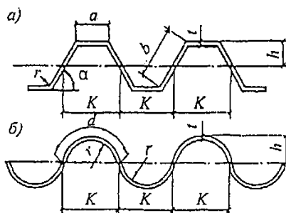
а - трапециевидный гофр; б - волнистый гофр
